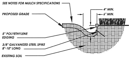
6 L2.0 LANDSCAPE EDGING DETAIL N.T.S.
